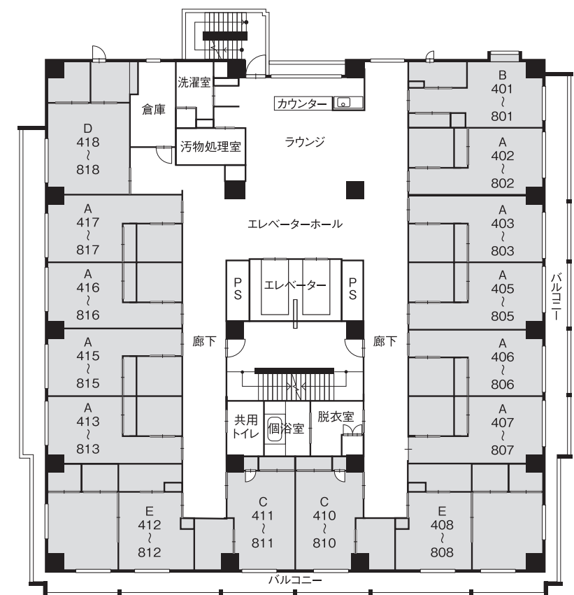
4～8階平面図
