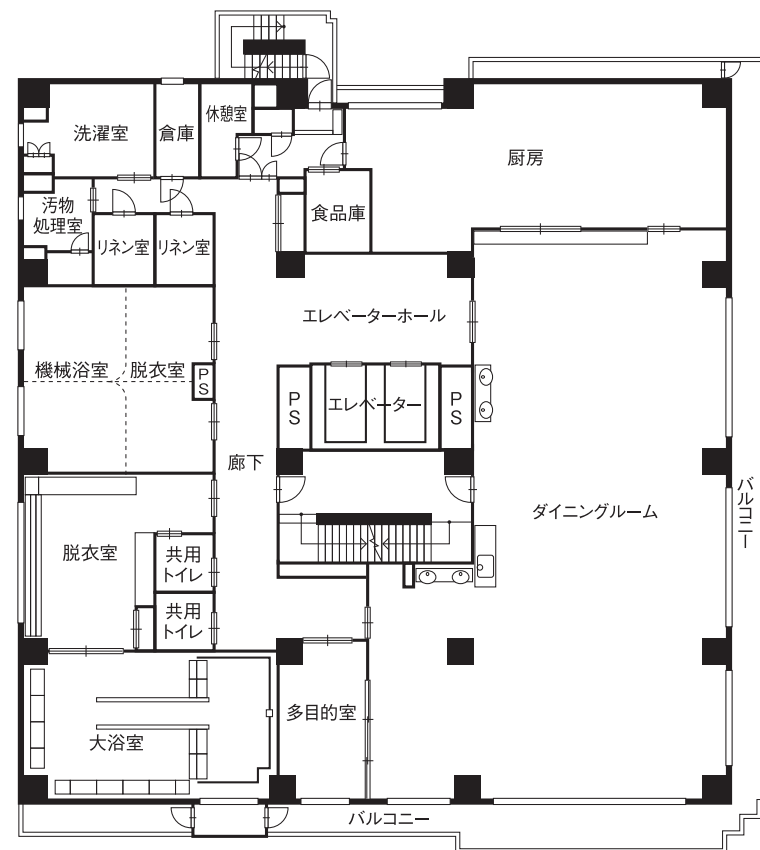
2階平面図
