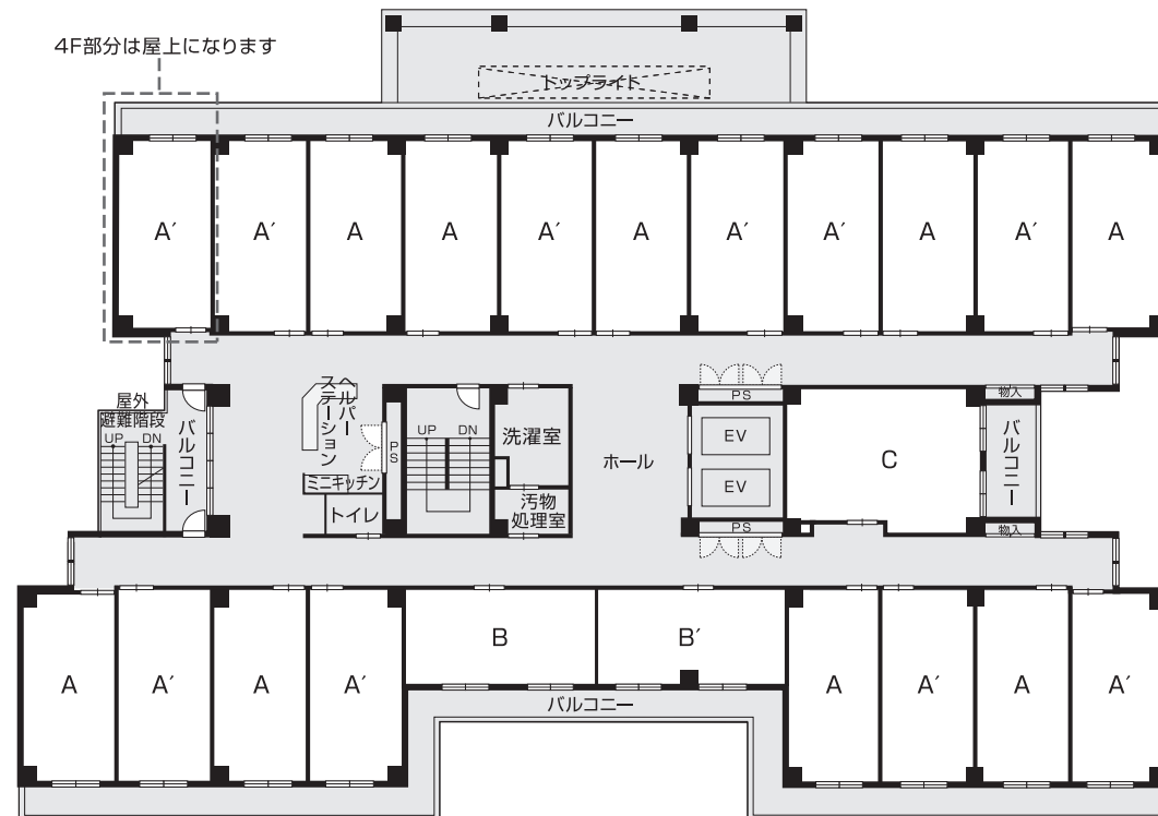
2階～4階平面図
