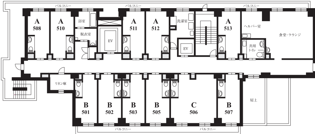
5階 平面図
