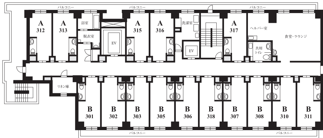
3階 平面図
