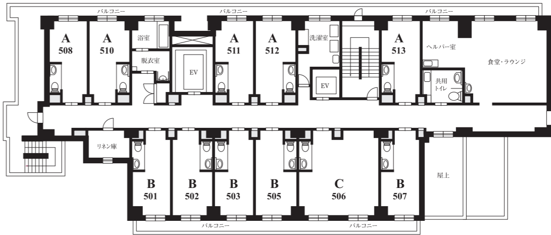
5階 平面図
