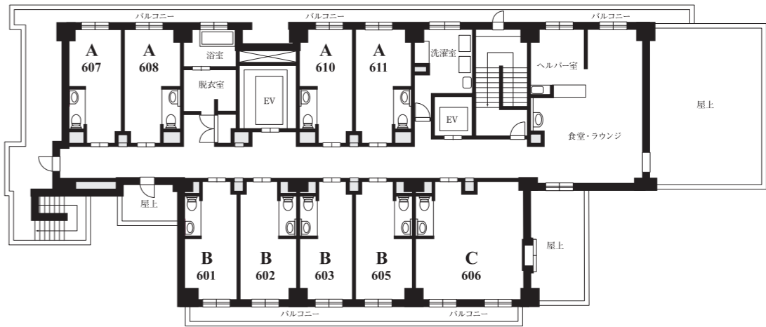
6階 平面図
