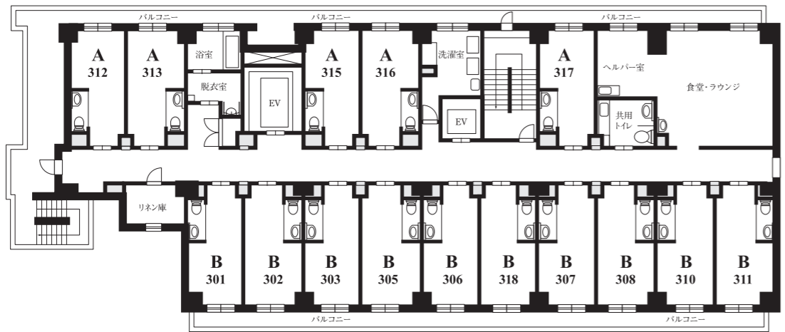
3階 平面図
